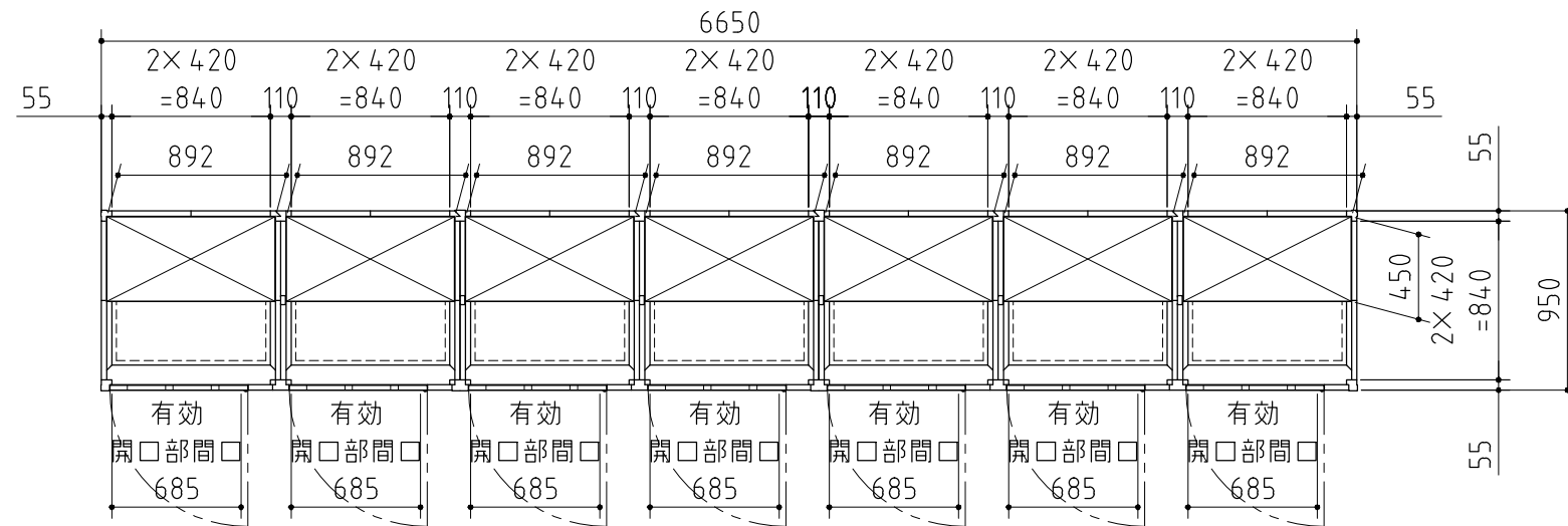
平面図
